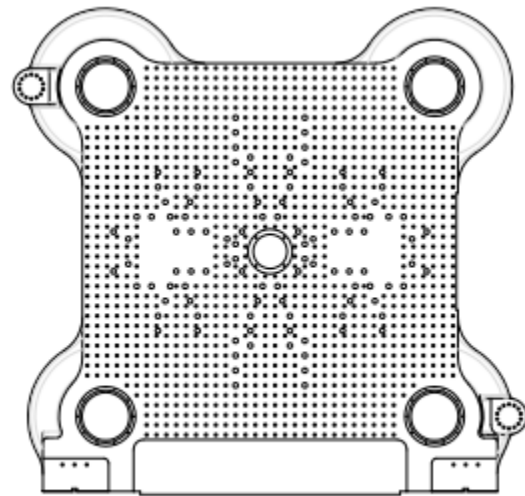
Moving Platen: Mold Side
