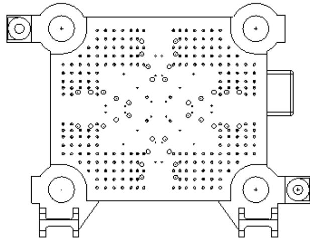
Moving Platen: Mold Side
