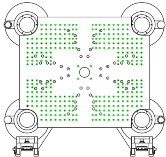
Moving Platen: Mold Side
