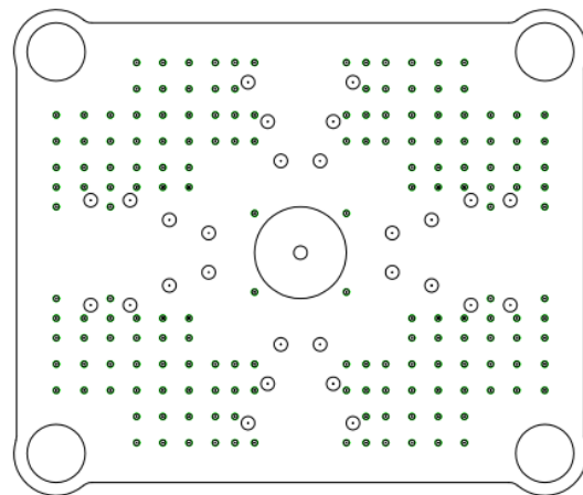
Moving Platen: Mold Side
