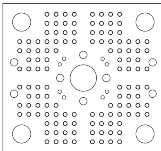
Moving Platen: Mold Side
